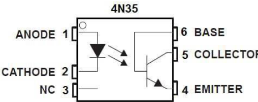
Fig.3. 4N35 Optocoupler pin layout
